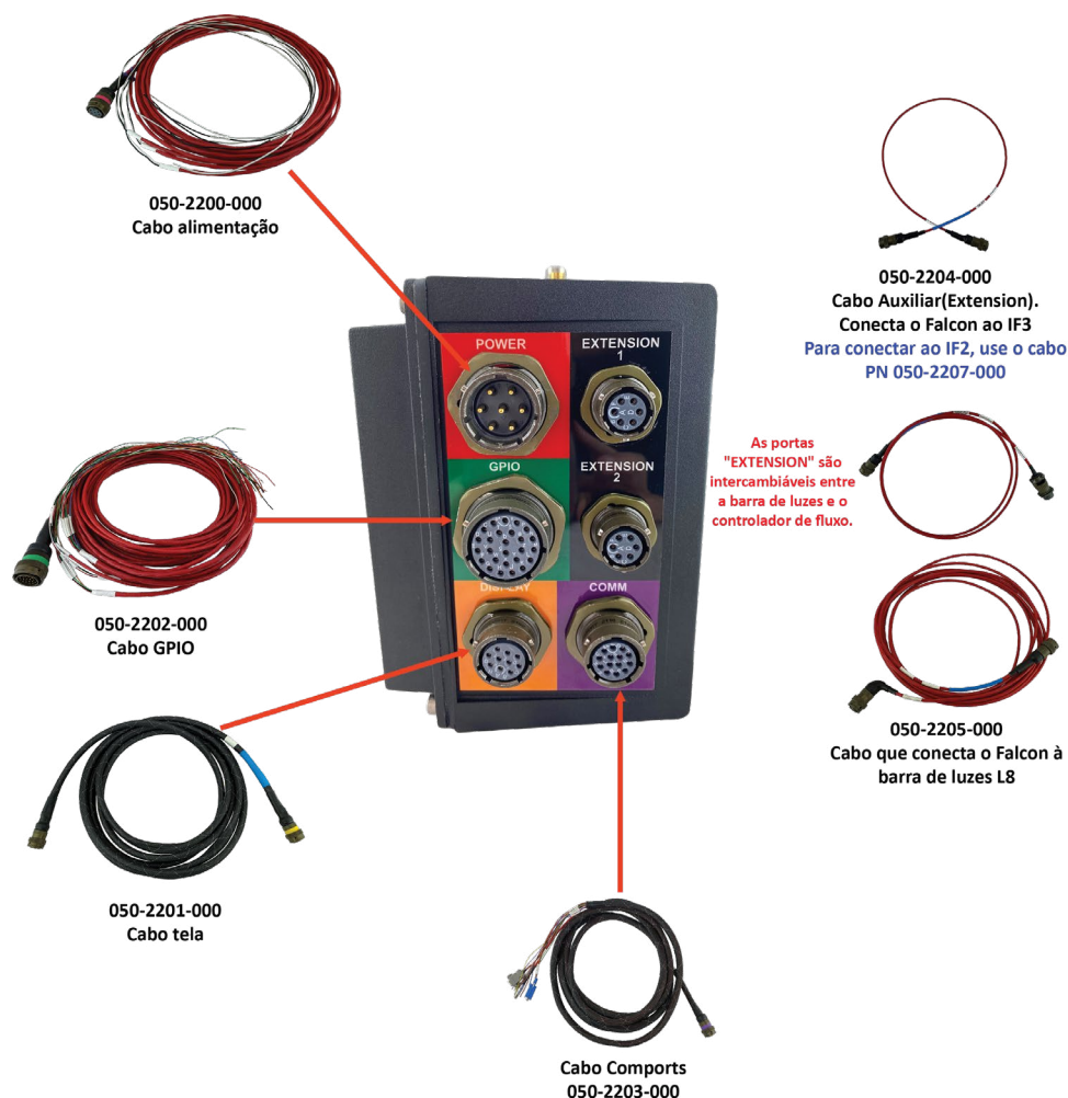
Figura 3-1: Conexões Frontais do Falcon
