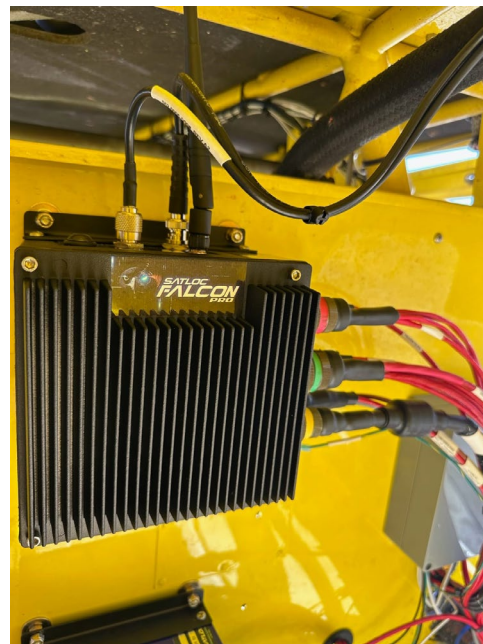
Figure 3-4: Imagem das conexões na parte superior do Falcon
