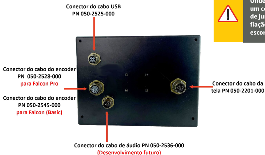
Figura 3-5: Conexões com a parte traseira da tela
