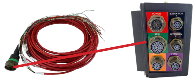
Figura 3-6: Conexão do cabo GPIO à CPU do Falcon
