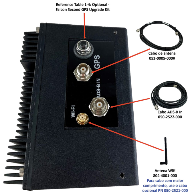
Figura 3-3: Conexões da parte superior do Falcon
