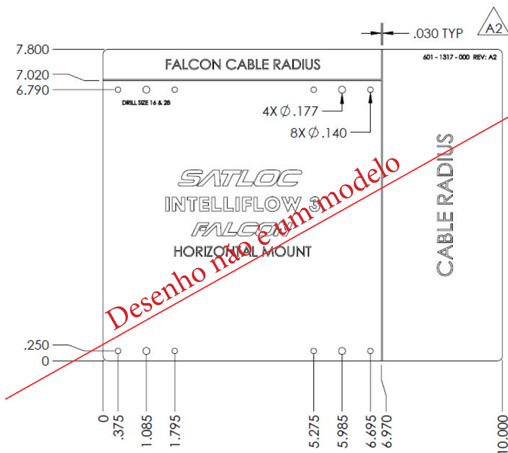
Dimensões para instalação Horizontal
