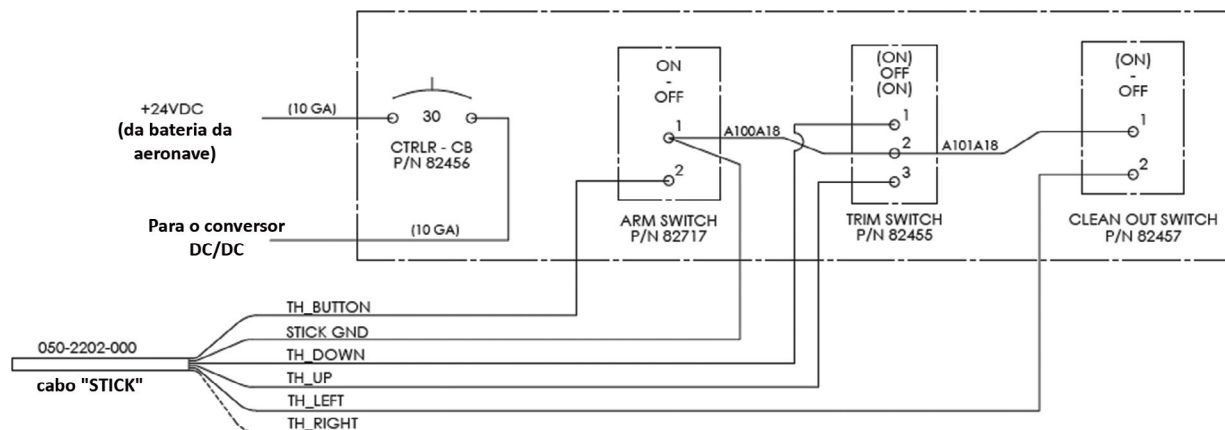
Figure 3-7: Conexões do cabo GPIO ao Transland Electric Gate
