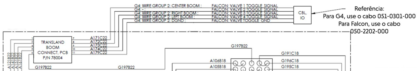
Figura 3-9: Esquema de fiação do Transland 50% ou 60% fechamento das válvulas da barra no painel de controle com o GPS Satloc
