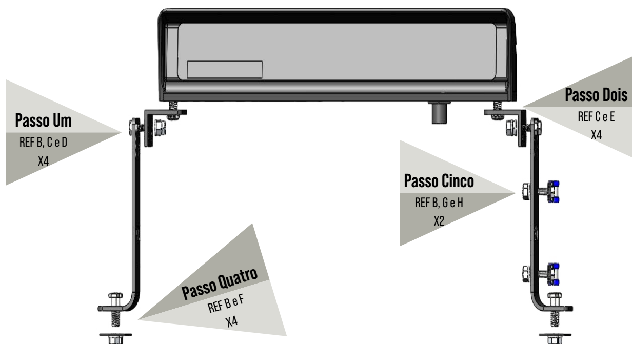
Figura 2-5: Vista Explodida da Montagem da Barra de Luzes L8
