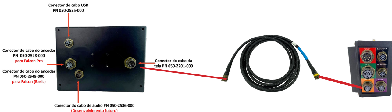
Figura 3-7: Conexões da Cabos da Tela
