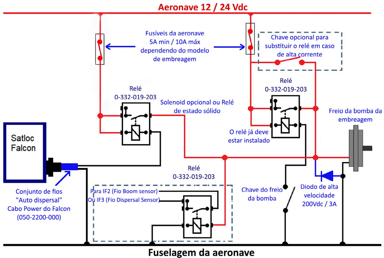
Figura 3-9: Diagrama de conexões dos cabos para aplicação automática
